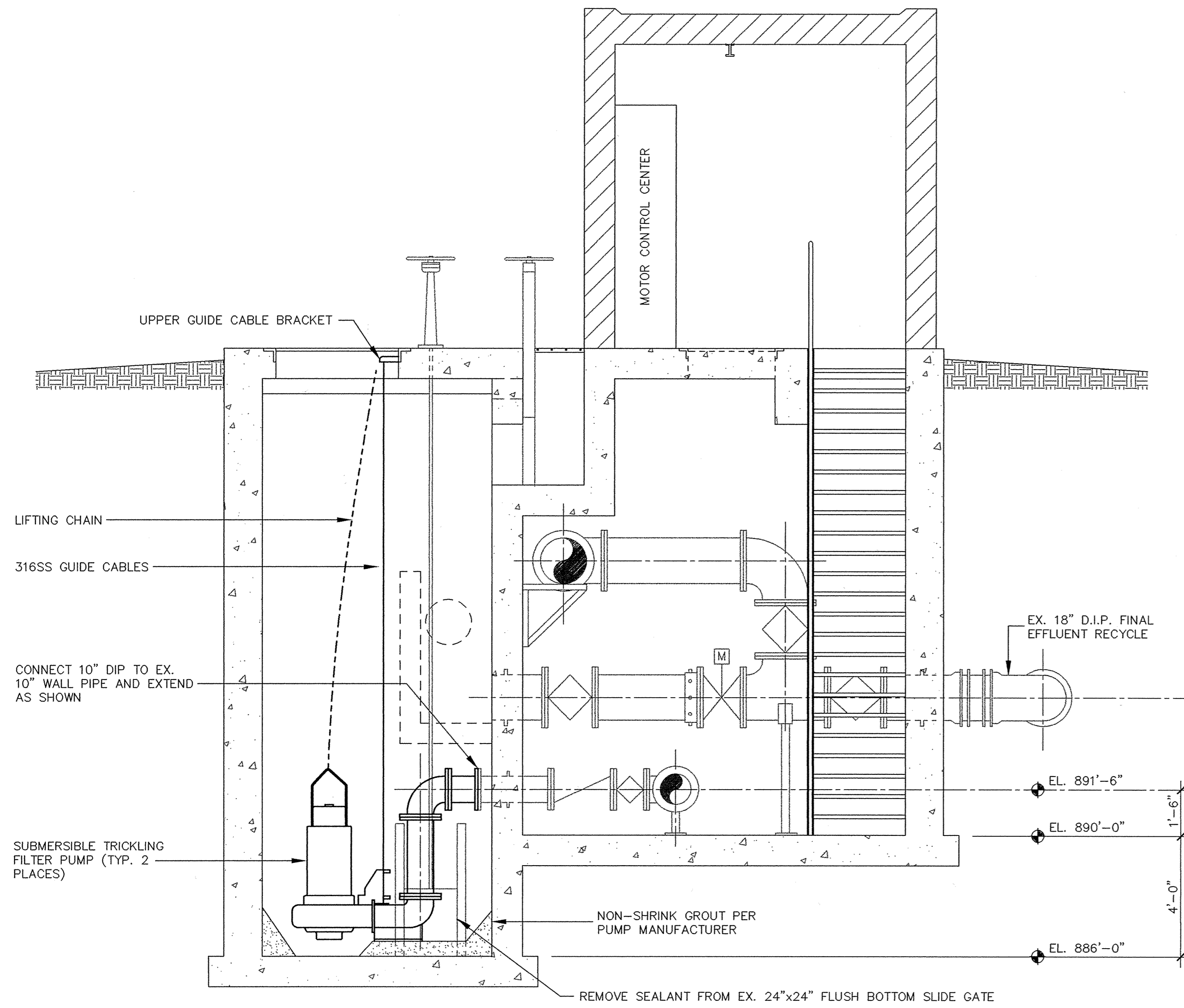
SECTION 1 Scale: 3/8" = 1'-0" P5
