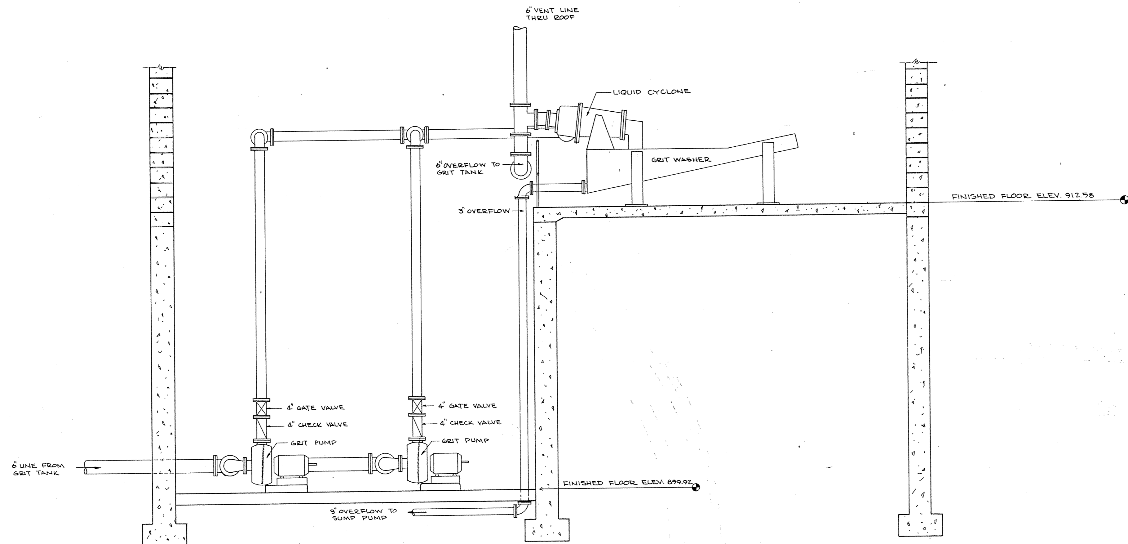
SECTION A SCALE: 3/8"=1'-0"
