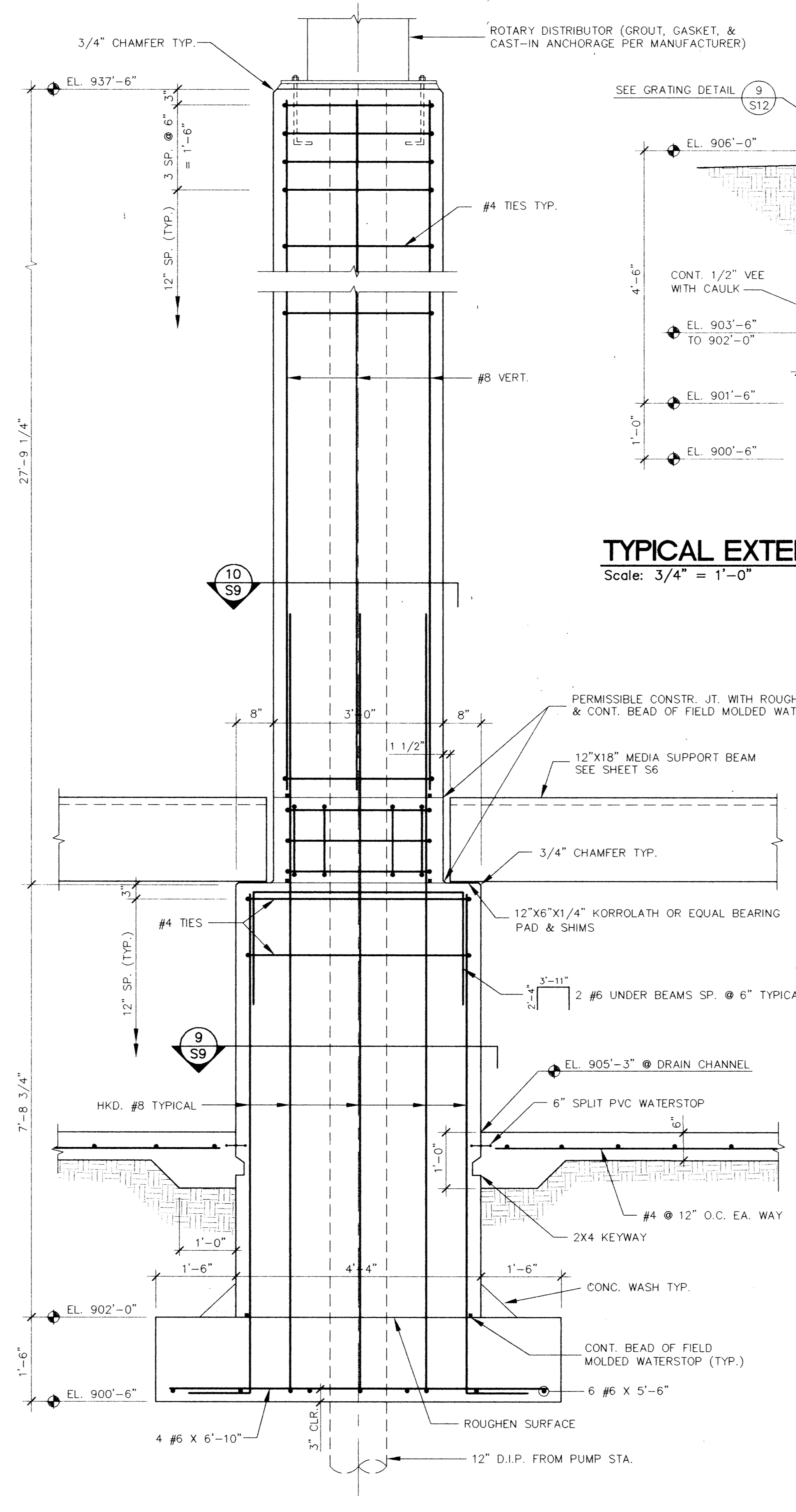
CENTER COLUMN SECTION 7 Scale: 3/4" = 1'-0" S9
