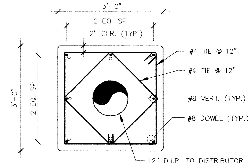
SECTION 10 Scale: 3/4" = 1'-0" S9
