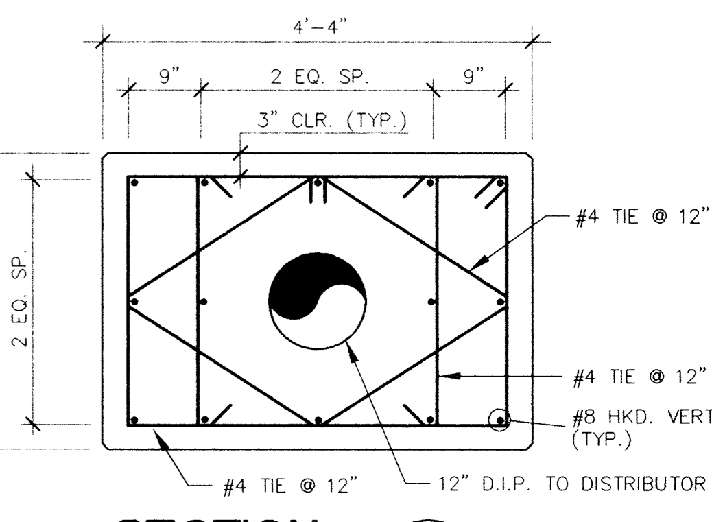
SECTION 9 Scale: 3/4" = 1'-0" S9
