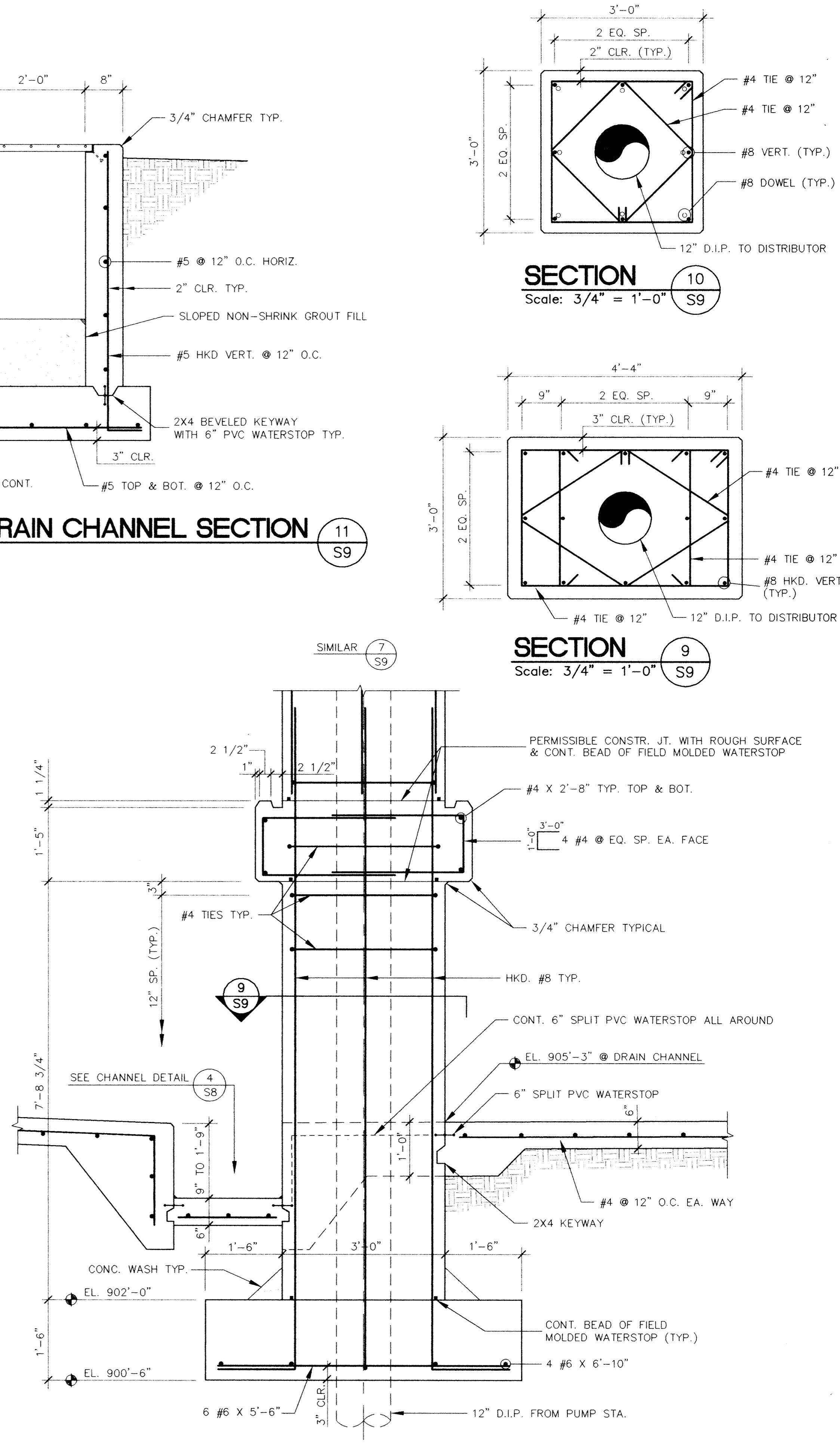
CENTER COLUMN SECTION 8 Scale: 3/4" = 1'-0" S9
