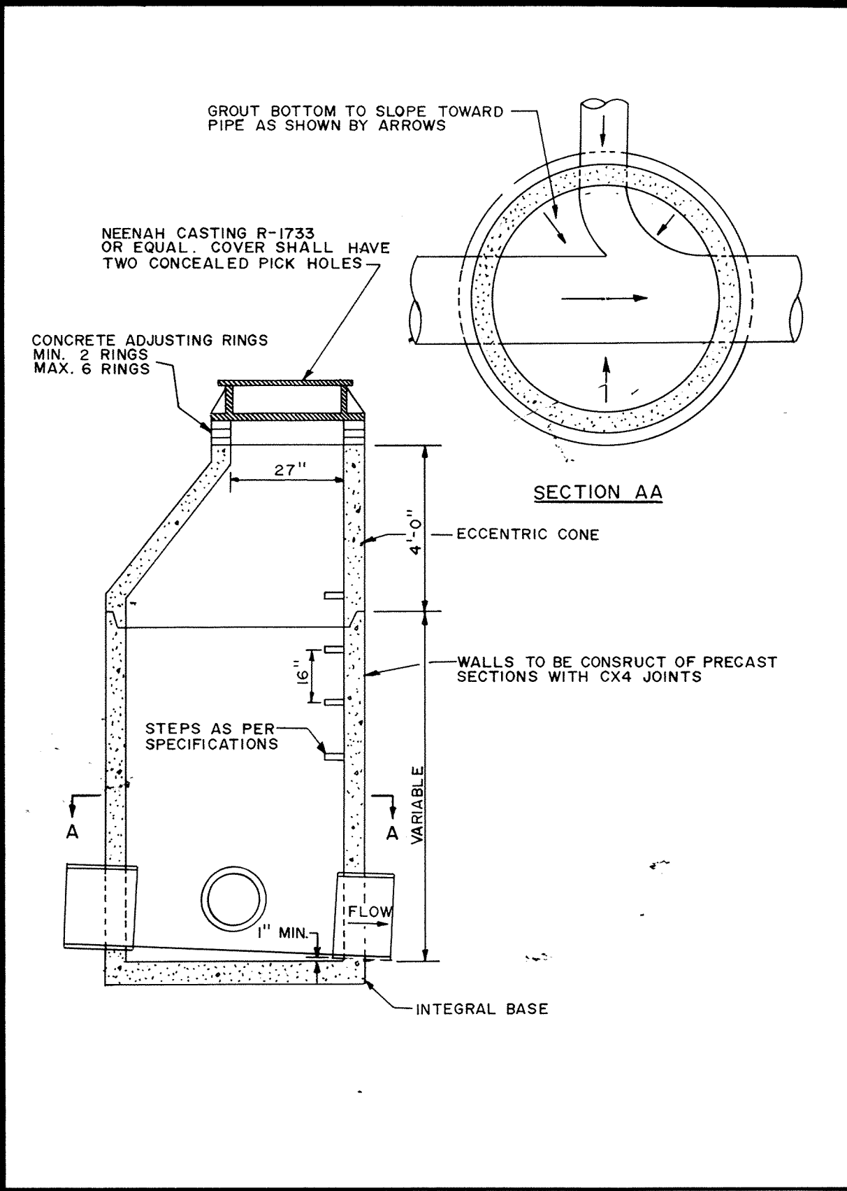
STANDARD MANHOLE
