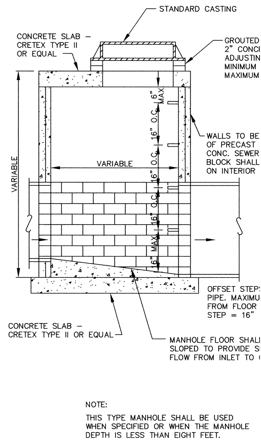
SLAB TOP MANHOLE
